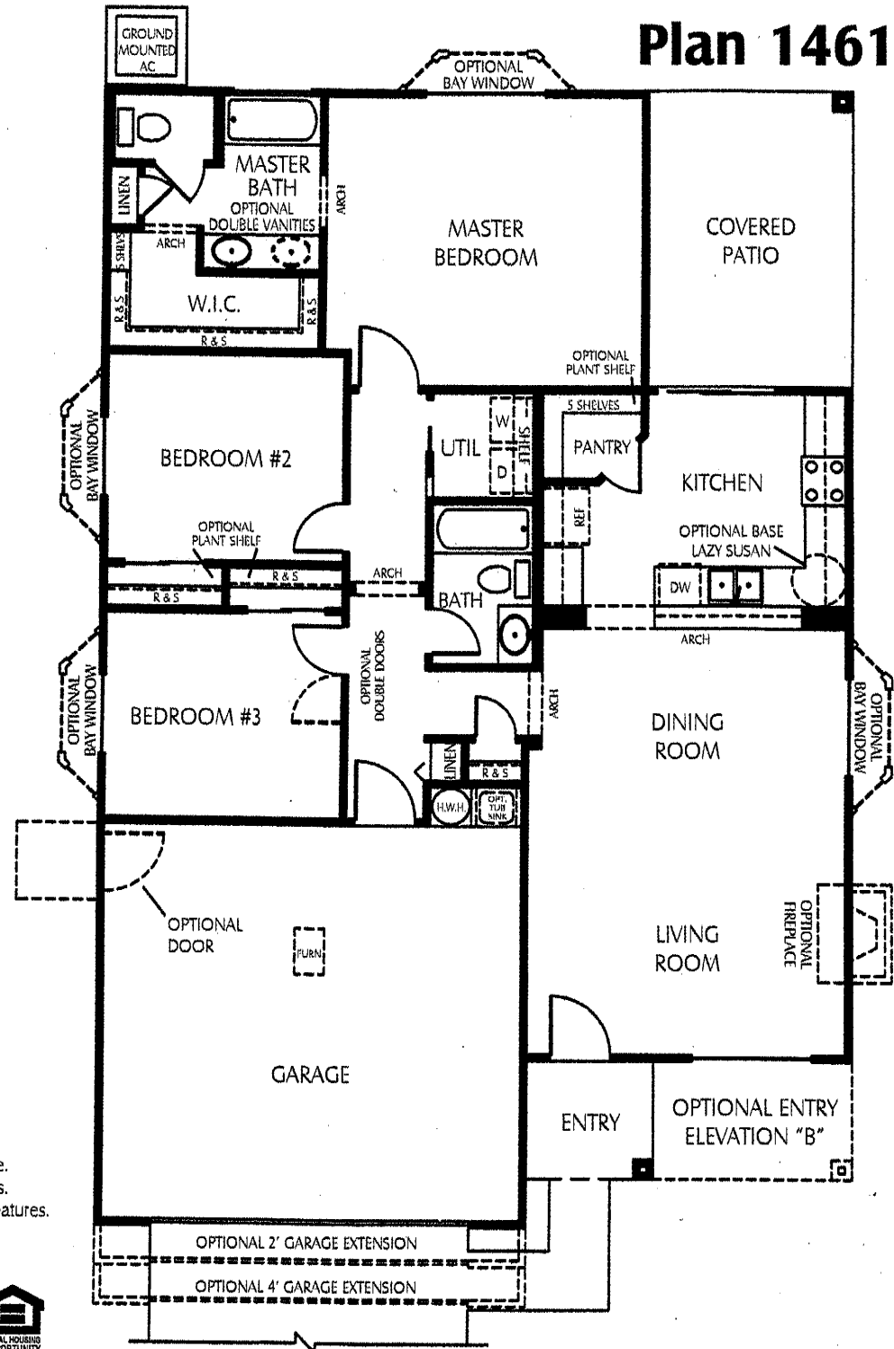
OPTIONAL FIREPLACE
